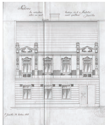
Původní plány na přestavbu Katolického domu z roku 1912
