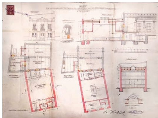
Plány Václava Tomišky z roku 1923 na přístavbu tělocvičny.
